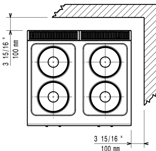
Boven aanzicht
